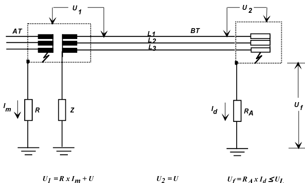
2 - Primeiro defeito na BT
