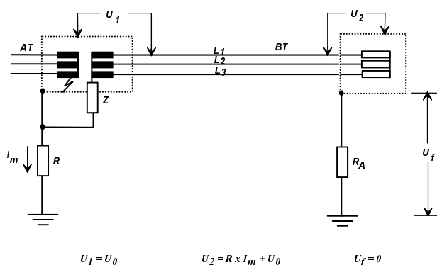
1 - Ausência de defeito na BT
