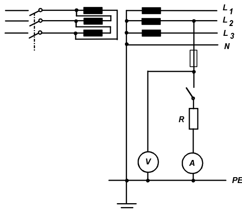
Figura D1 — Método das quedas de tensão
