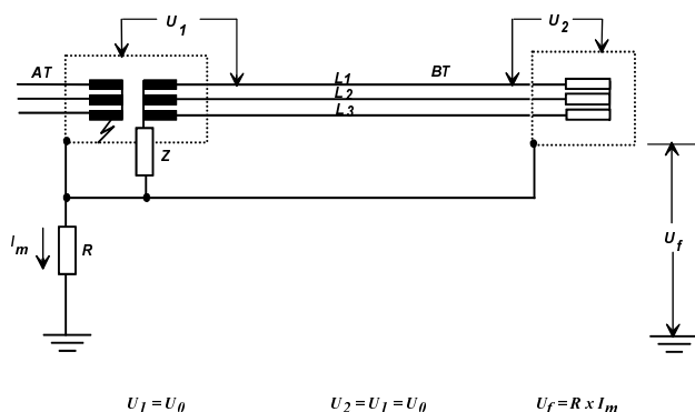
1 - Ausência de defeito na BT
